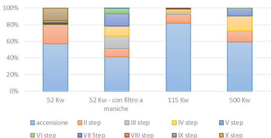
Grafico 2 - Emissioni di Idrocarburi Policiclici Aromatici nelle diverse fasi della combustione
